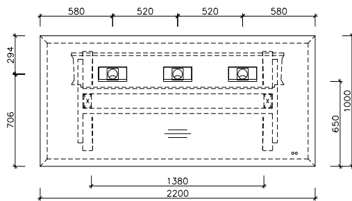
U 09 + U 10 Table
