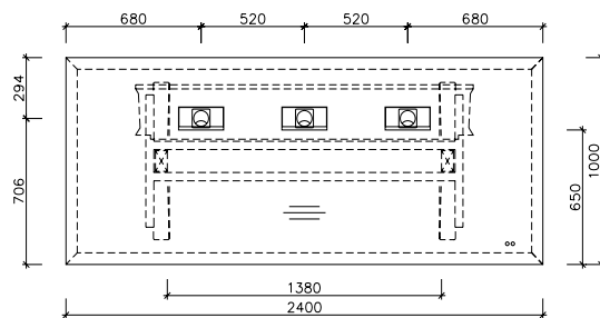
U 11 + U 12 Table
